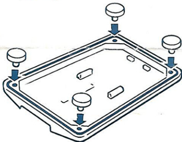
Abb. 1 Einsetzen der Gummifüße
