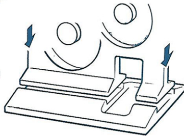
Abb. 2 Befestigen von Basis und Aufbau
